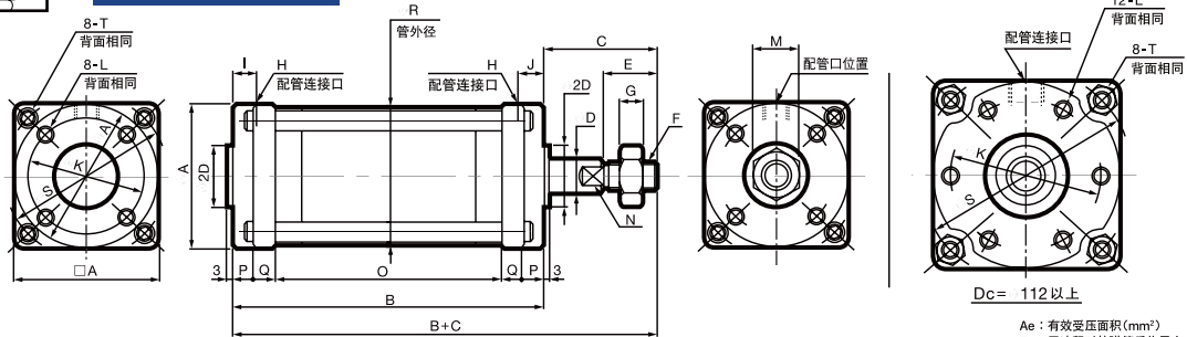
■ FCS/SCS 型基本尺寸表
