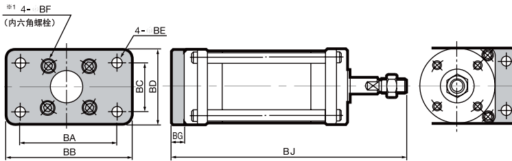
后法兰型尺寸图
