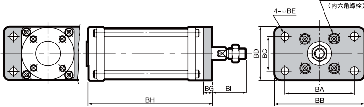
前法兰型尺寸图
