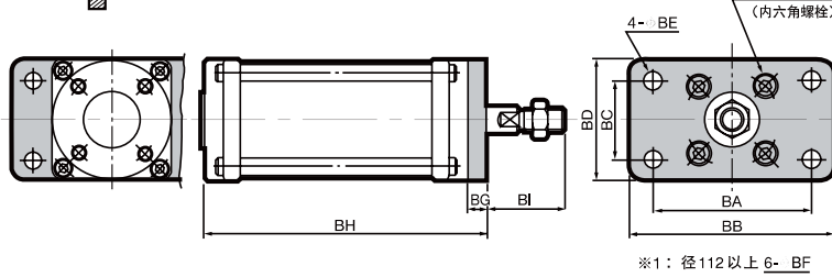
前法兰型尺寸图
