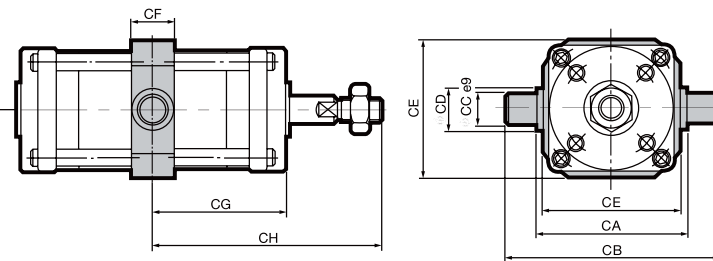
轴销型尺寸图
