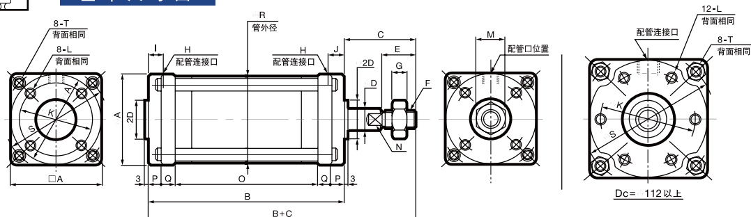
■ FCD/SCD型基本尺寸表
